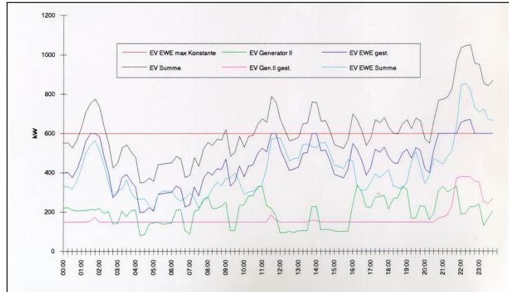
Diagramm Eigenenergieerzeugung/Netzbezug
