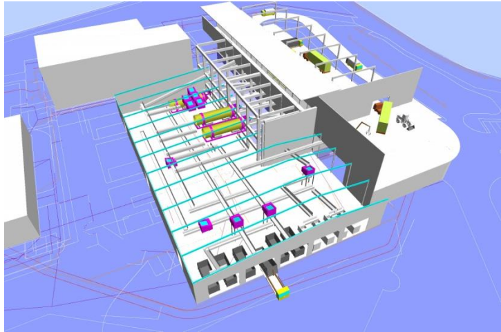
Anlagenkonzept Vorschaltanlage
